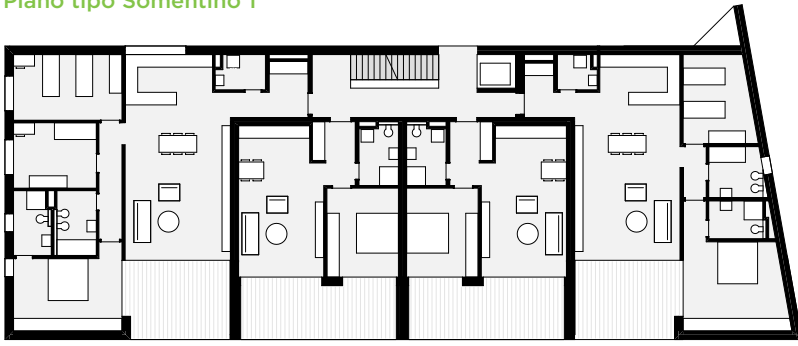
Piano tipo Somentino 1
