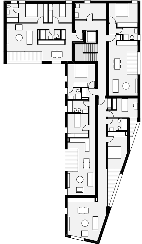
Primo e secondo piano
